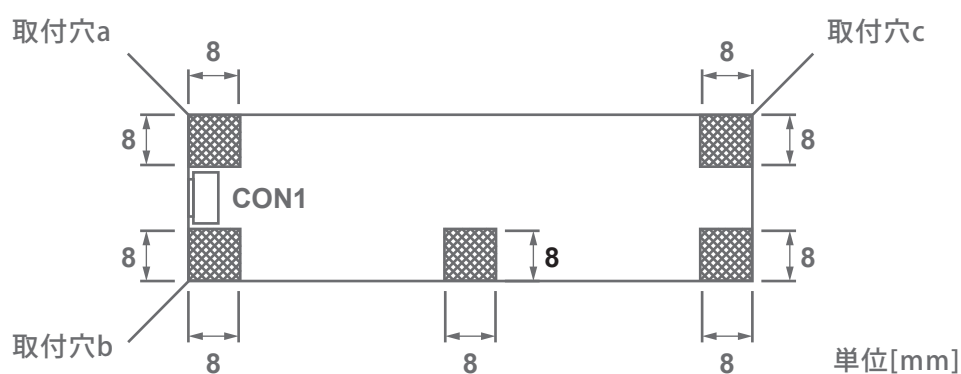
UOHC3240 | 取り付け金属部の許容範囲
